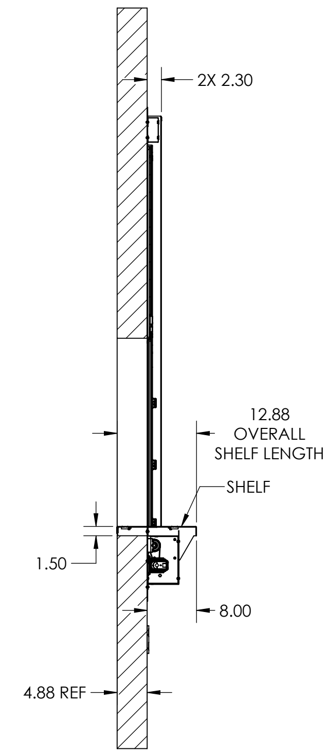
SECTION A-A
